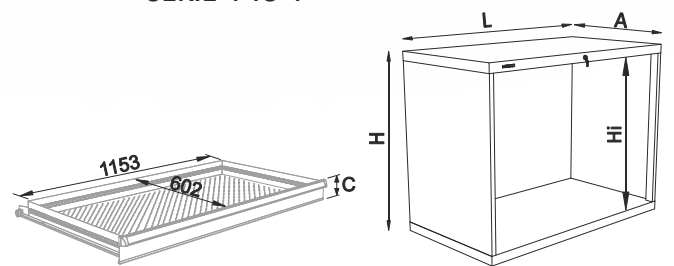
SERIE 143 1
